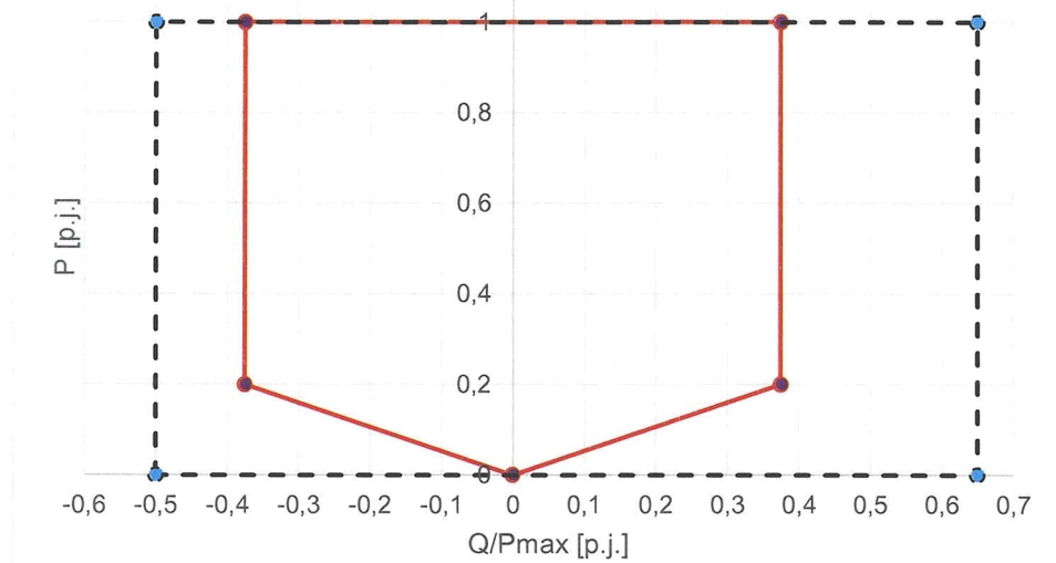
Obr. 3 Diagram dodávky jalového výkonu při nižší než maximální dodávce činného výkonu pro nesynchronní výrobní moduly kategorie D
